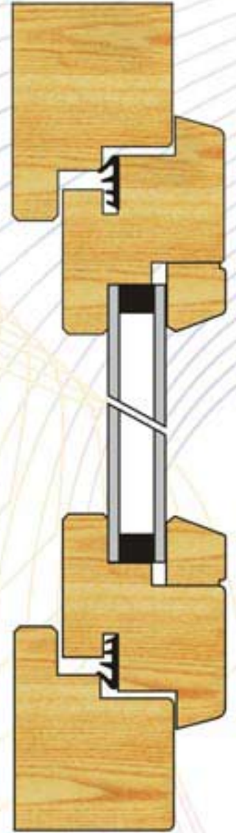
B KESİTİ
