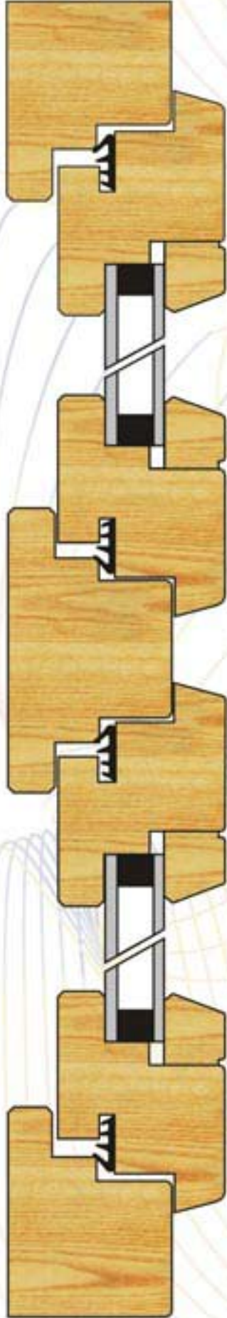
A KESİTİ
